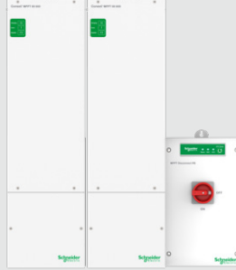
2 MPPT 80/100 600 con RS de desconexión de MPPT
