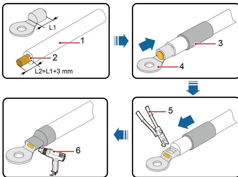
Figura 5-2 Engaste del terminal OT
