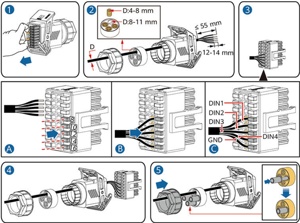
Figura 5-30 Instalación del cable
