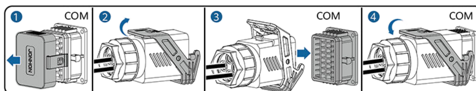
Figura 5-28 Fijación del conector del cable de señal
