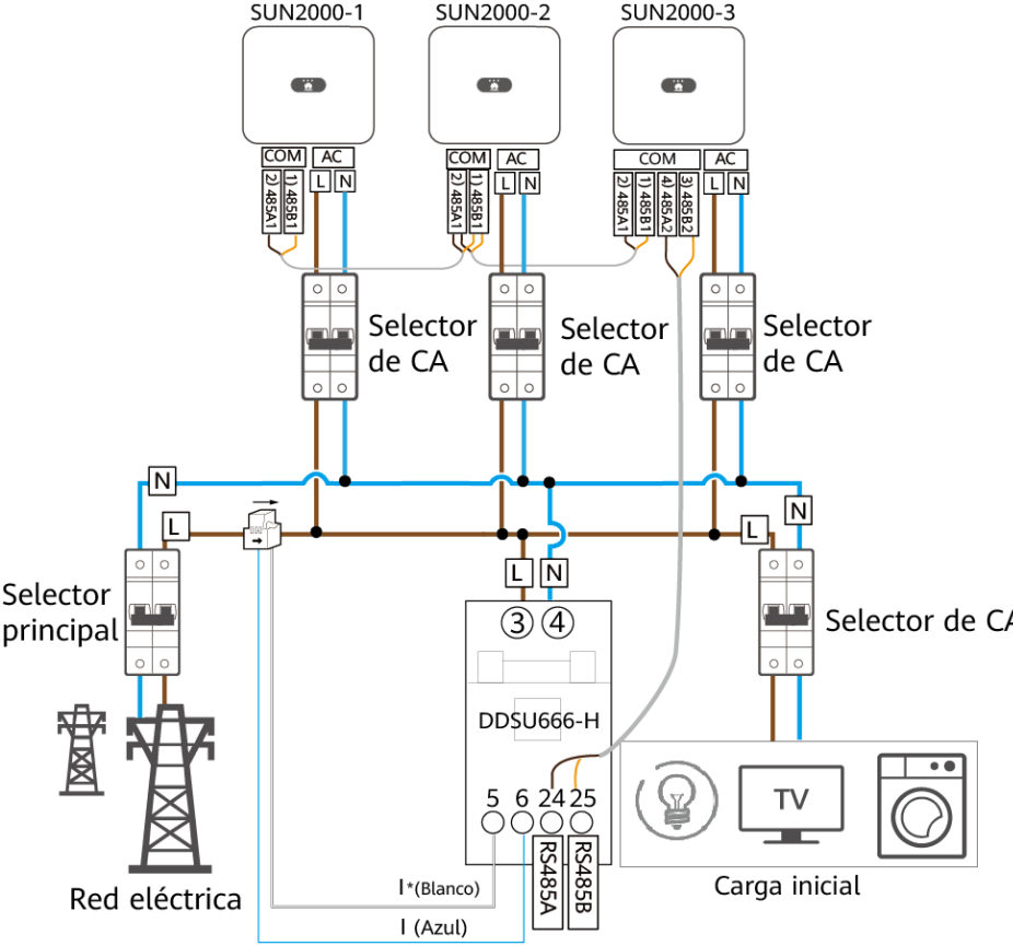
Figura 5-22 Conexión de los cables al sensor de energía inteligente (conexión a la red en fase)
