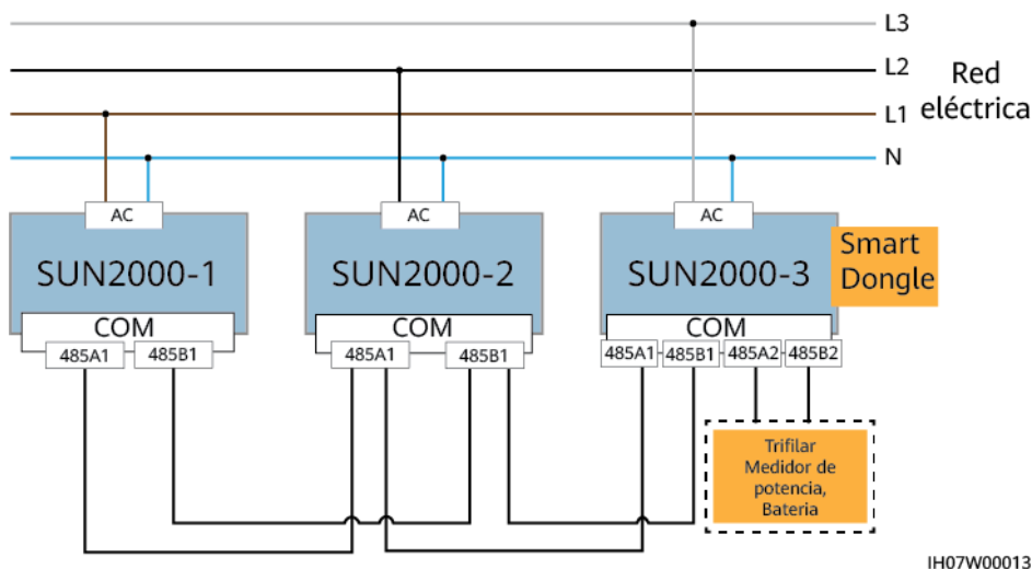
Figura 5-23 Conexión a la red trifásica equilibrada
