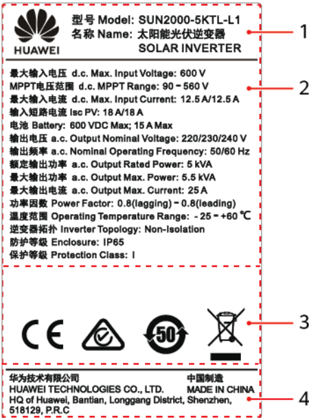
Figura 2-6 Placa de identificación (SUN2000-5KTL-L1 como ejemplo)
