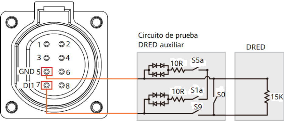
Figura 7-19 Diagrama de cableado de la función DRM
