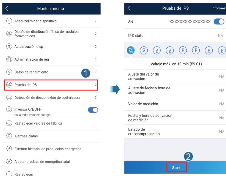
Figura 7-18 Prueba de IPS
