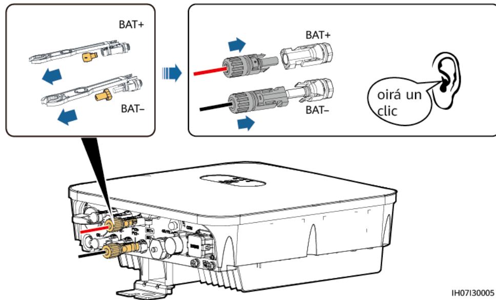
Figura 5-17 Conexión de los cables de la batería
