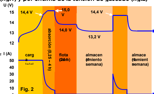
Curvas de carga: hasta la tensión de gaseado (fig.1) y por encima de la tensión de gaseado (fig.2)
