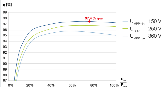
PIKO MP plus 1.5-1
