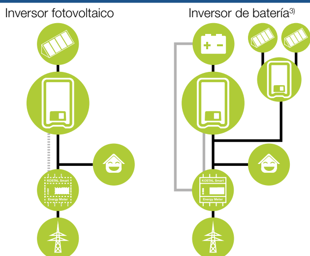
PIKO MP plus 1.5 hasta 3.6 con 1 seguidor PMP
