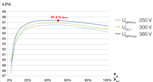
PIKO MP plus 1.5 hasta 3.6 con 1 seguidor PMP
