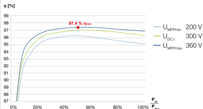
PIKO MP plus 2.0-1
