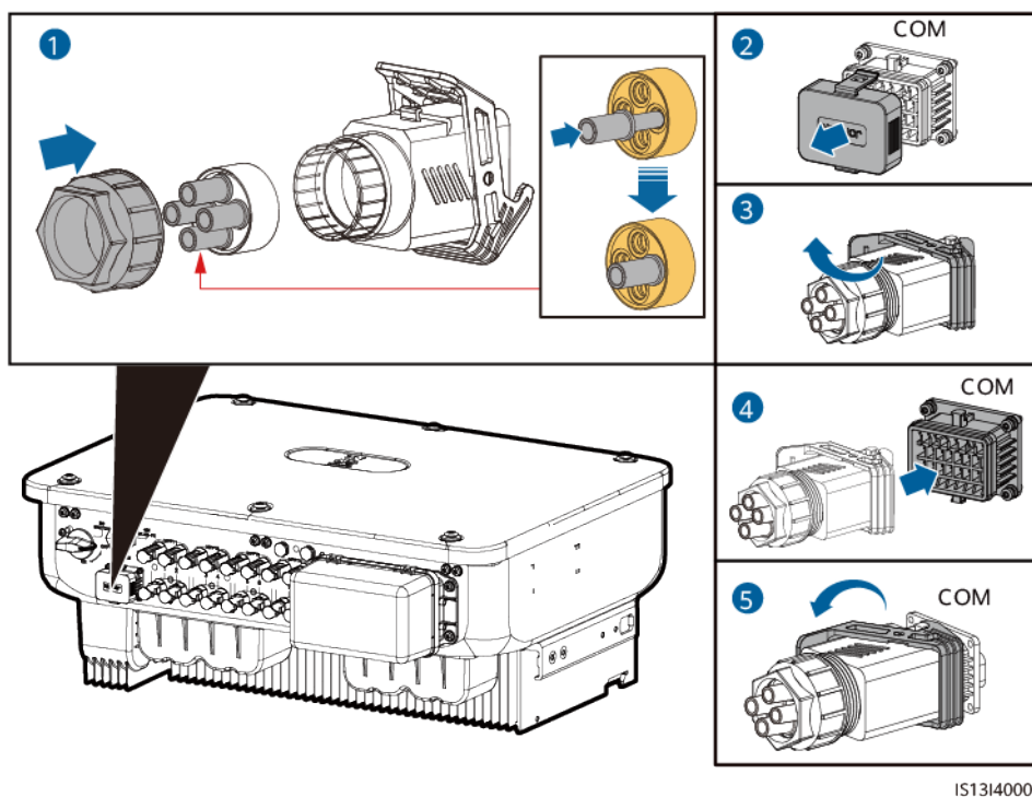
Figura 5-16 Fijación del conector del cable de señal
