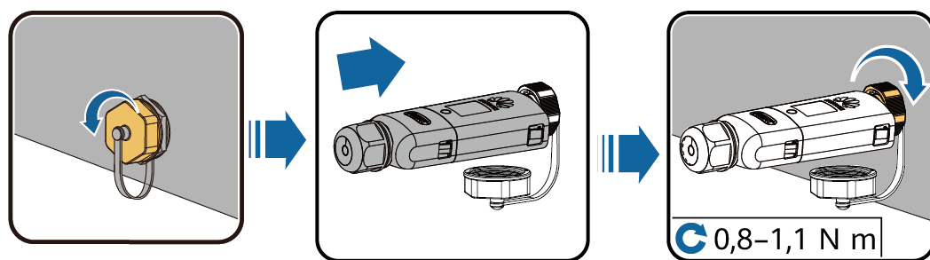
Figura 5-13 Instalación del Smart Dongle WLAN-FE (comunicación WLAN)
