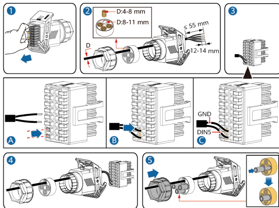
Figura 5-26 Cómo instalar el cable
