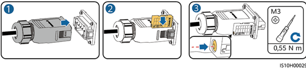
Figura 5-10 Cómo asegurar el conector de CA
