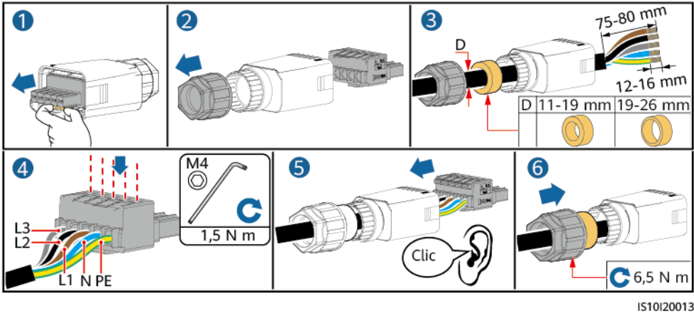
Figura 5-9 Cable de cinco conductores (L1, L2, L3, neutro y conexión a tierra)
