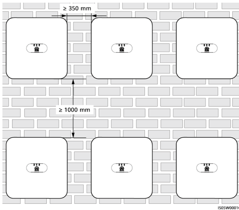
Figura 4-5 Instalación apilada (no recomendada)
