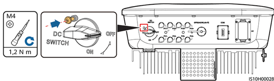
Figura 8-1 Instalación del tornillo de bloqueo del interruptor de CC
