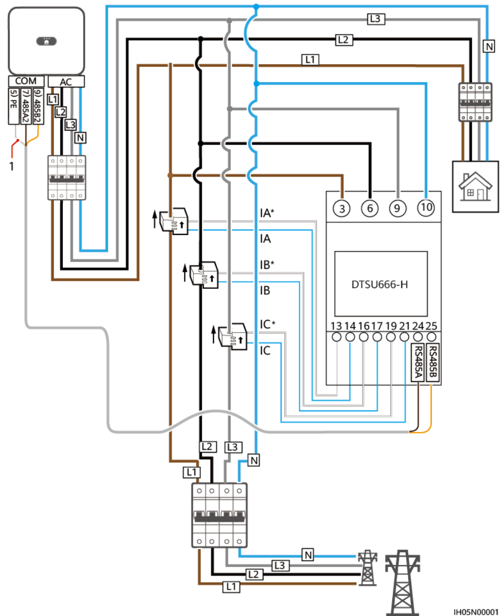
Figura 5-23 Conexión de cable (cuatro hilos, trifásico)
