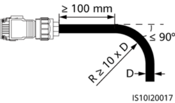
Figura 5-11 Recorrido de los cables
