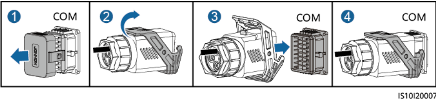
Figura 5-30 Cómo ajustar el conector del cable de señal
