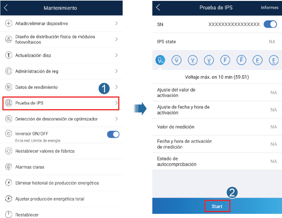
Figura 7-13 Prueba de IPS
