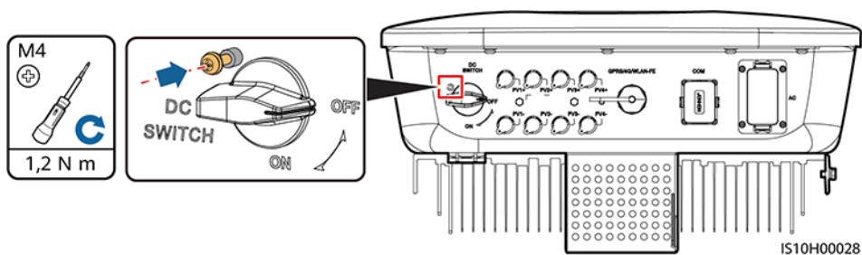
Figura 4-10 Instalación del tornillo de bloqueo del interruptor de CC
