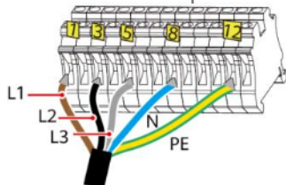
Terminal del lado de la Backup Box de reserva (trifásico)
