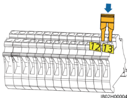
Borne de CA del inversor X3 (trifásico)
