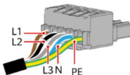
Terminal del lado del inversor (trifásico)
